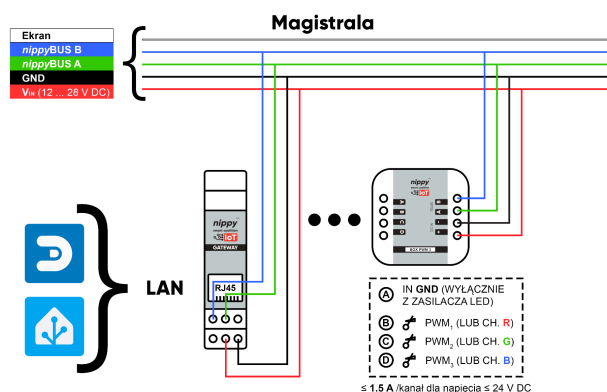
Uproszczony schemat połączeń Smart Home nippy™ z modułem nippy™ BOX LED Dimmer 3 PWM (rys.1)
