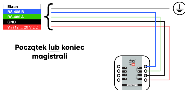
Schemat podłączenia modułu nippy™ BOX LED Dimmer 3 PWM na początku lub końcu magistrali (rys.3)
