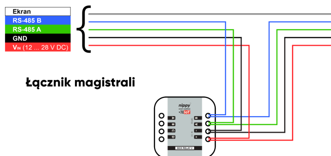
Schemat podłączenia modułu nippy™ BOX LED Dimmer 3 PWM jako łącznika magistrali (rys.4)
