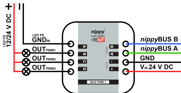
Schemat wyprowadzeń modułu nippy™ BOX LED Dimmer 3 PWM (rys.2)
