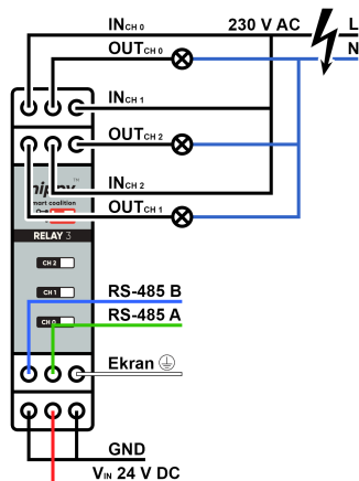
Schemat wyprowadzeń modułu nippy™ DIN Relay 3 dot. sterowania 230V AC (rys.3)
