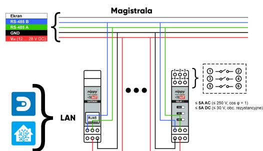
Uproszczony schemat połączeń Smart Home nippy™ z modulem nippy™ DIN Relay 3 (rys.1)
