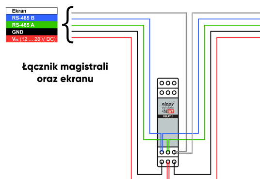
Schemat podłączenia modułu nippy ™ DIN jako łącznika magistrali oraz ekranu (rys.6)
