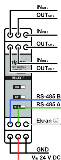
Schemat wyprowadzeń modułu nippy™ DIN Relay 3 (rys.2)
